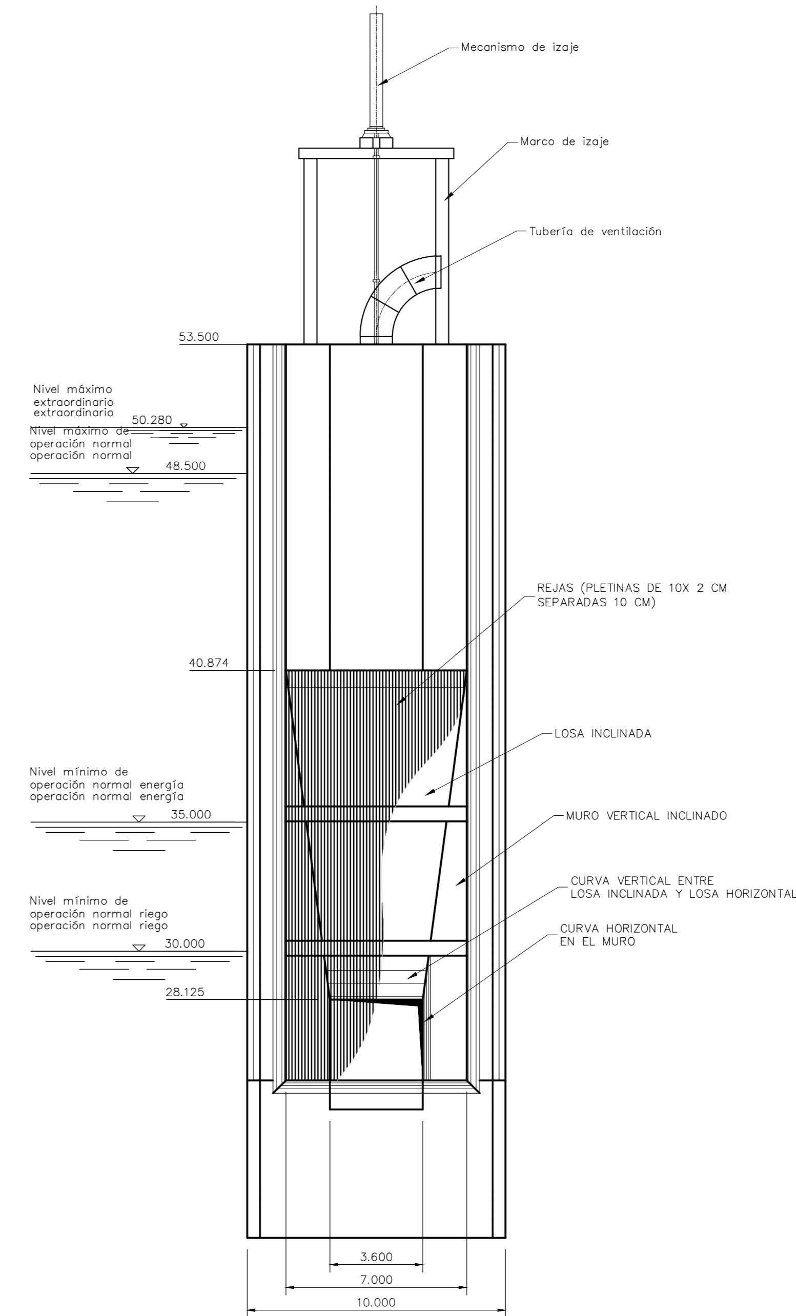
VISTA FRONTAL DE LA TOMA DE AGUAS Escala: 1:150
