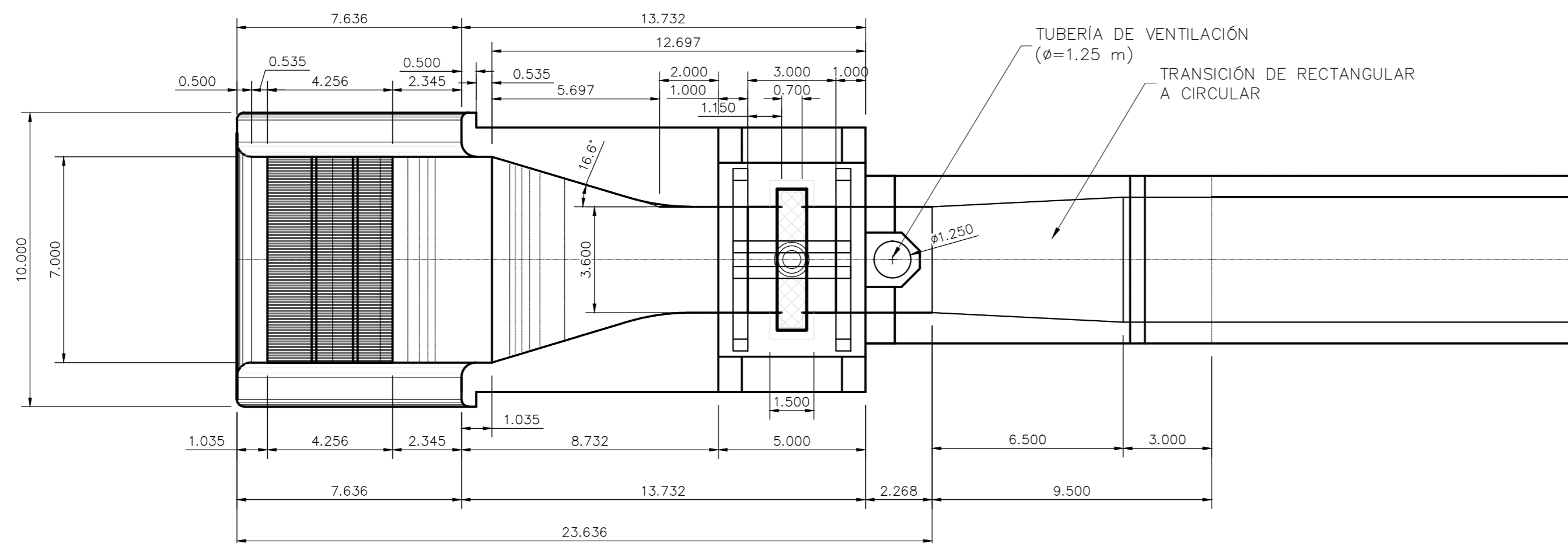
VISTA EN PLANTA EN DETALLE DE LA TOMA DE AGUAS Escala: 1:150
