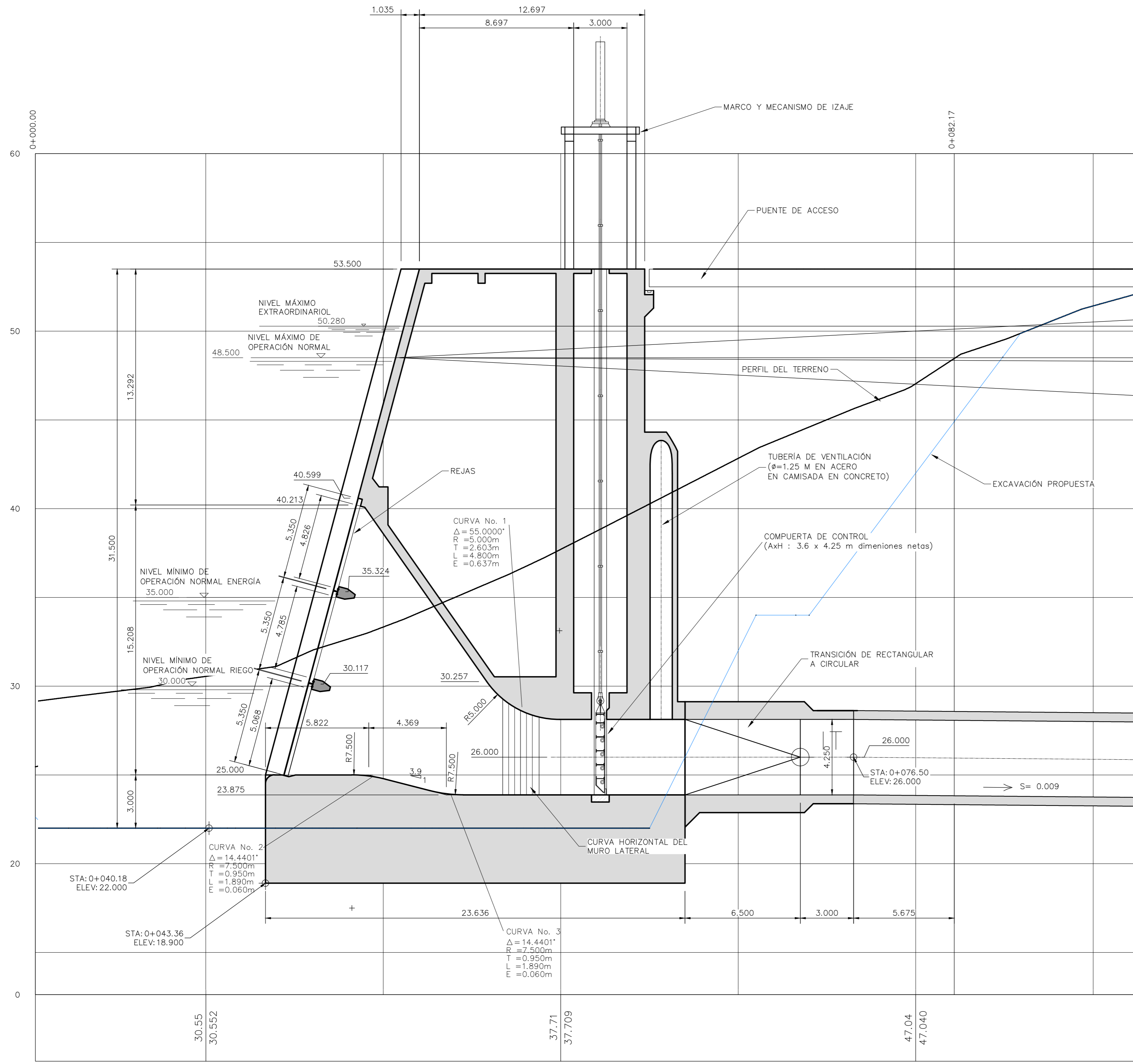
PERFIL LONGITUDINAL DE DETALLE DE LA TOMA DE AGUAS Escala: 1:150
